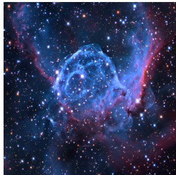
Casque de Thor (Nébuleuse)
