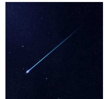
Étoile filante
