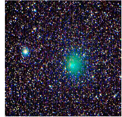
Comète d'Encke
