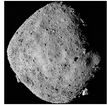
Astéroïde
