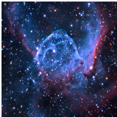
Coque de Thor (Nébuleuse)
