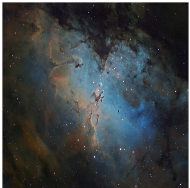
Nébuleuse de l'Aigle
