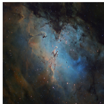
Nébuleuse de l'Aigle
